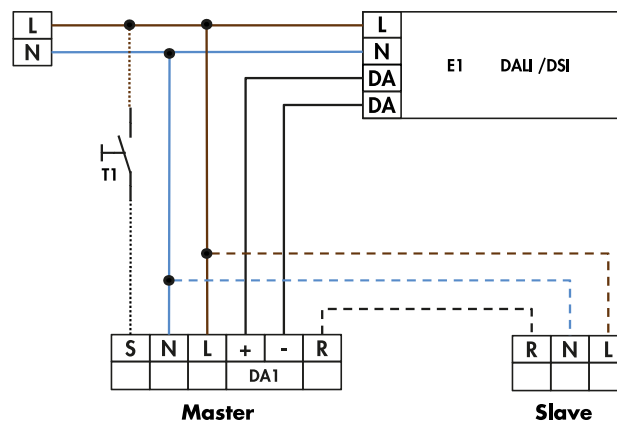
Schaltbild
